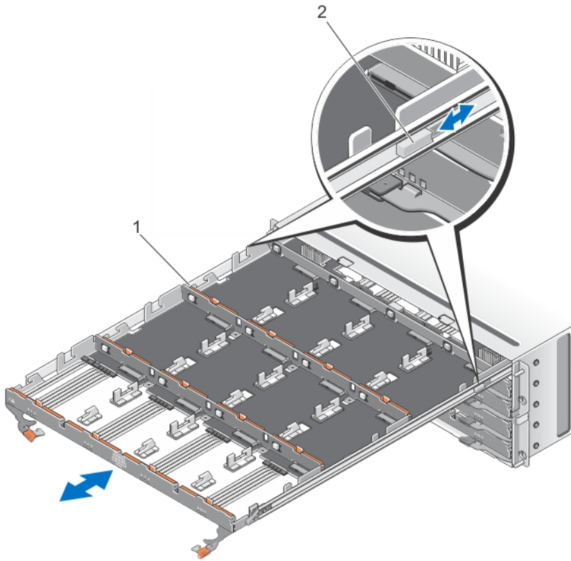
图 13: 卸下和安装物理磁盘盘位
