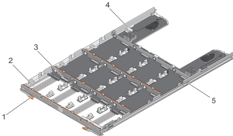
图 11: 物理磁盘盘位内部
