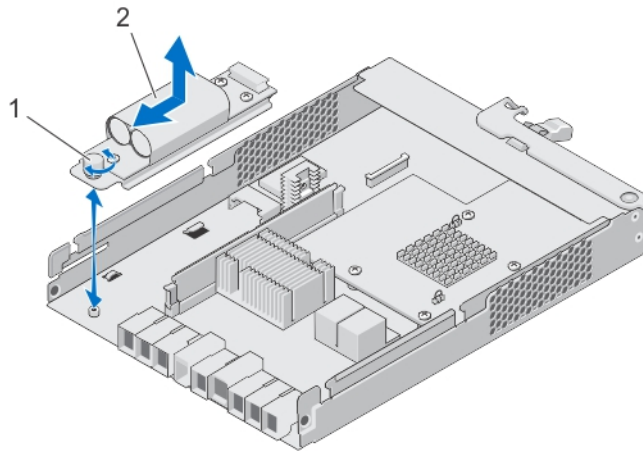
图 22: 卸下和安装 RAID 控制器模块备用电池装置
