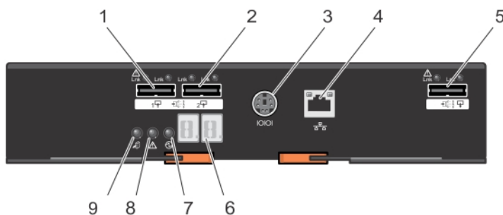
图 9: MD3060e 扩展模块部件和指示灯
