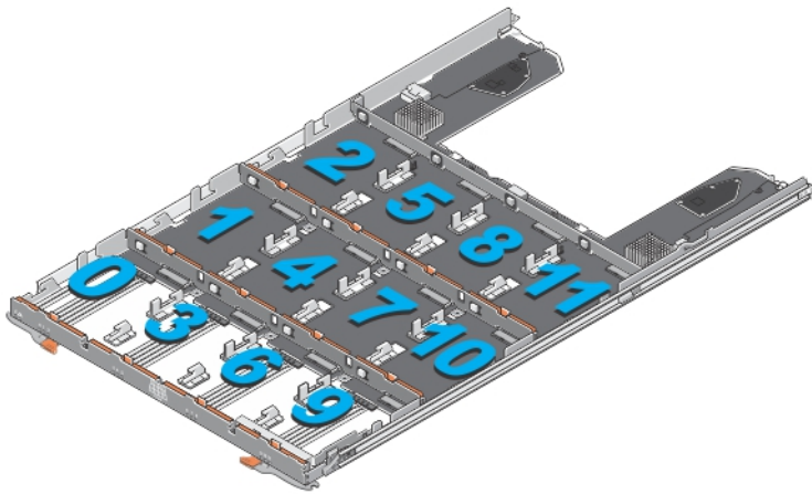
图 14: 物理磁盘盘位上的插槽编号
